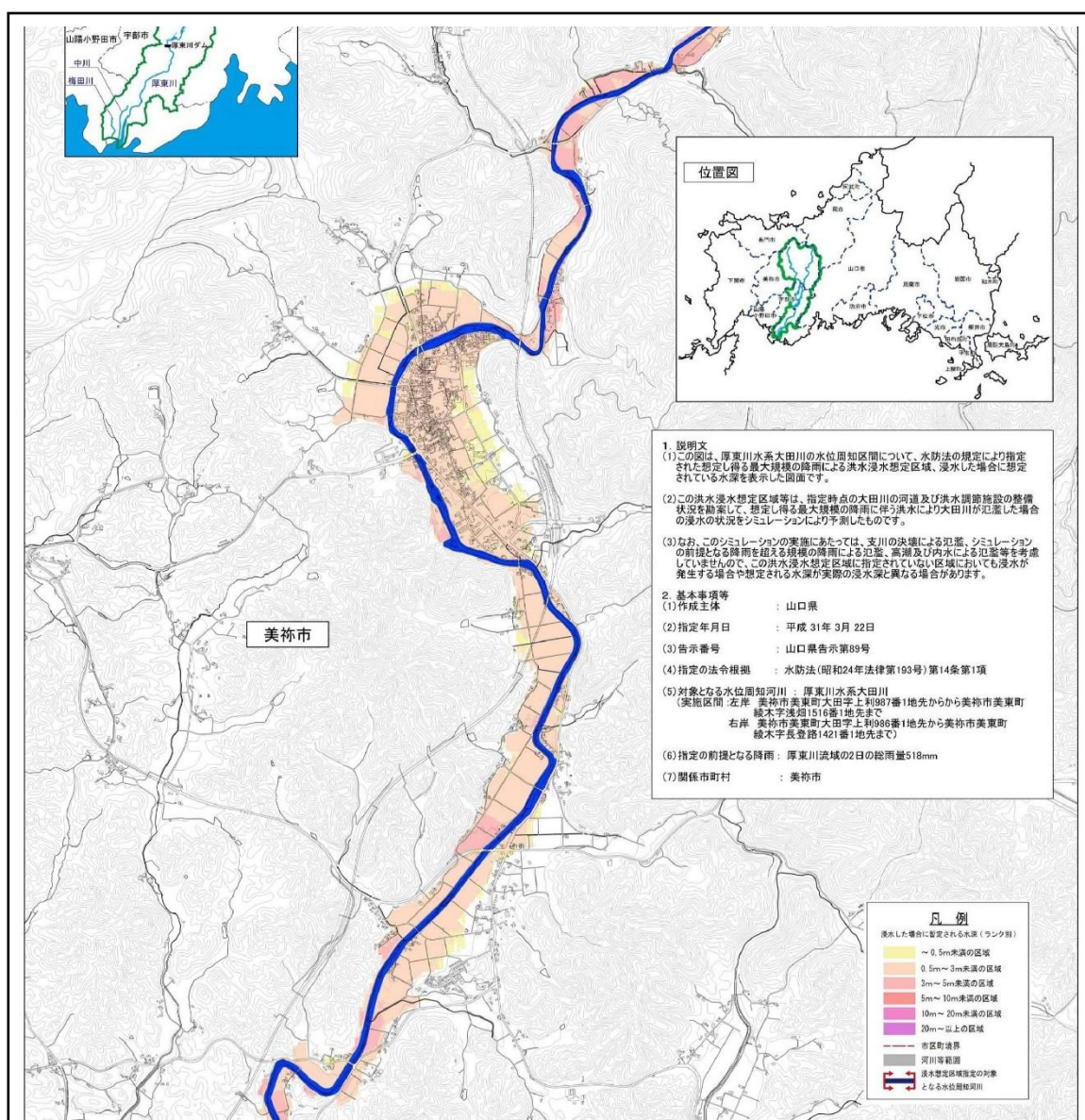
(図-資2) 厚東川水系大田川洪水浸水区域図[想定最大規模]
