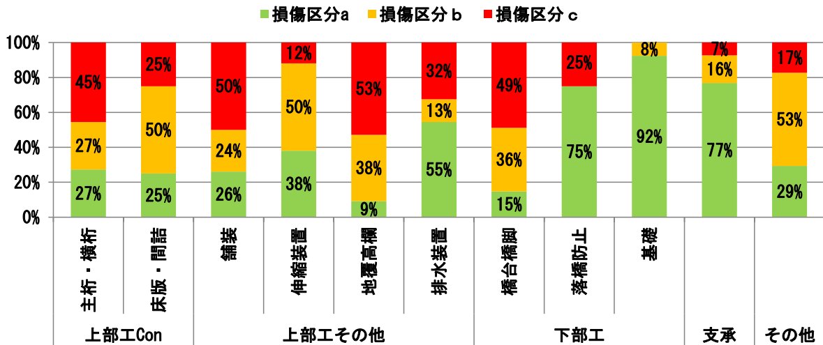
図2-6 PC橋の部材区分別の損傷区分の割合
