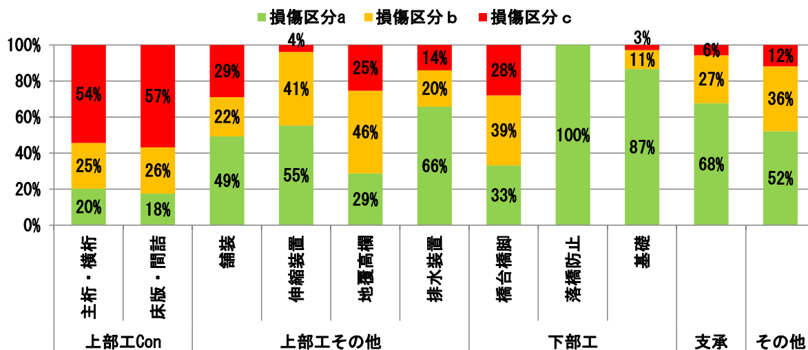
図2-5 RC橋の部材区分別の損傷区分の割合
