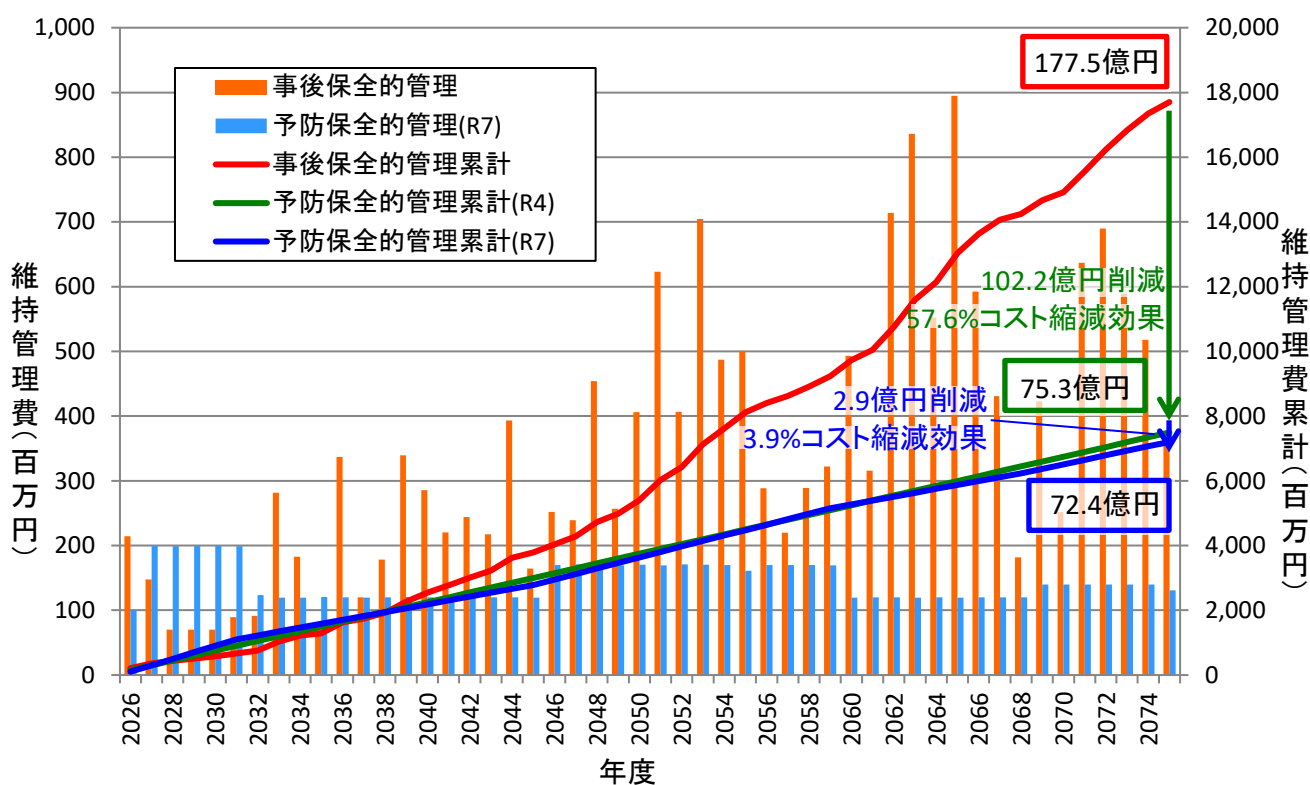
図5-1 計画によるコスト縮減効果の試算結果
