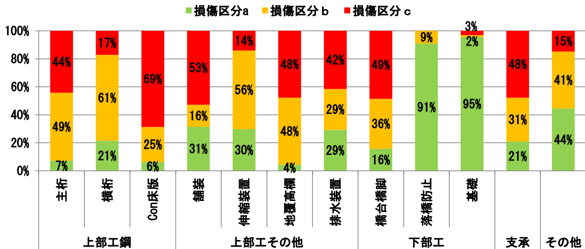
図2-7 鋼橋の部材区分別の損傷区分の割合
