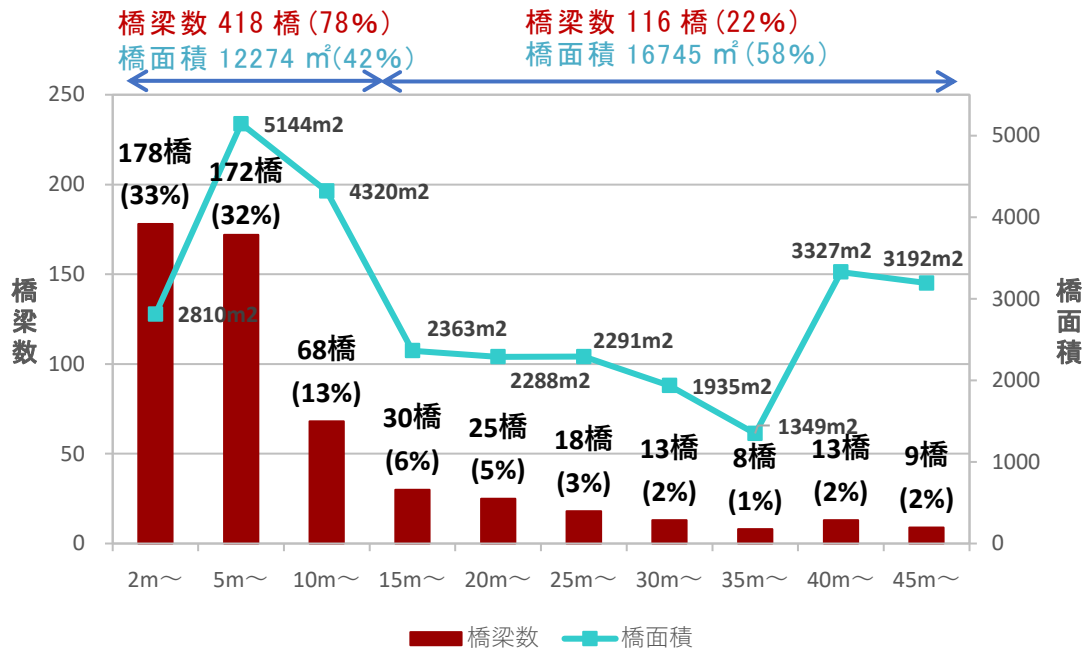
図2-2 橋長ごとの橋梁数及び橋面積
