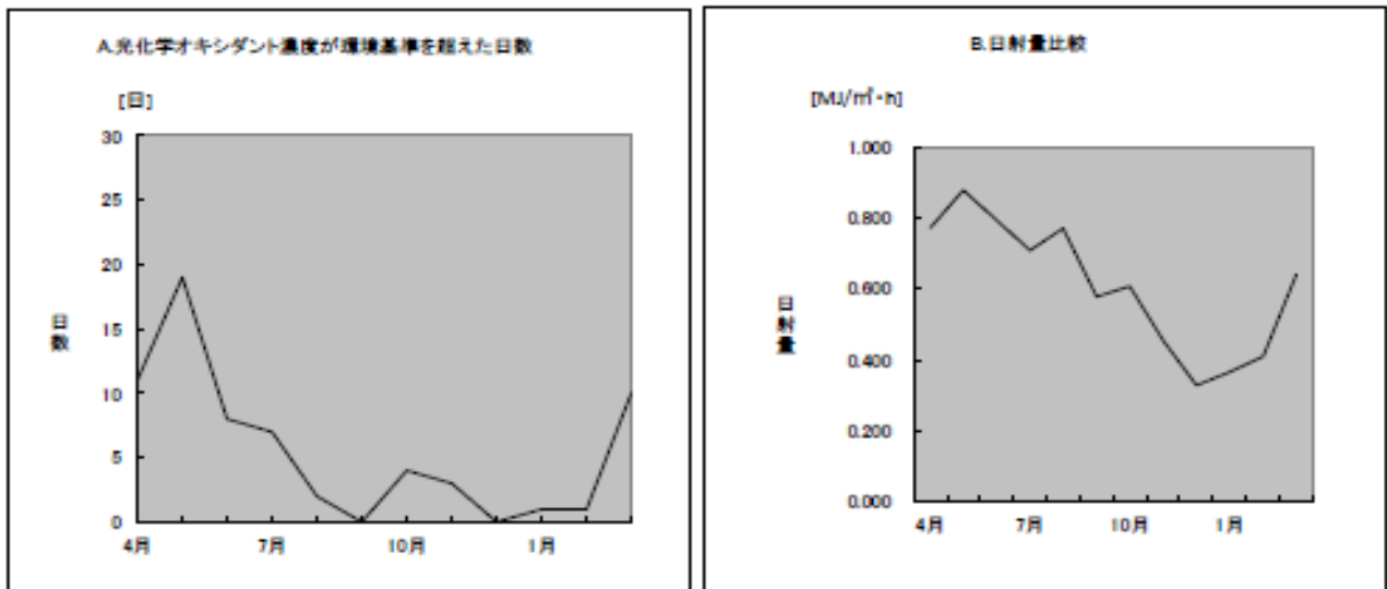
図3-6 光化学オキシダント濃度が環境基準を超えた日数
