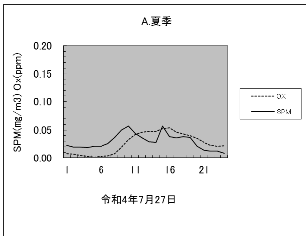
図3-3 浮遊粒子状物質濃度の日変化
