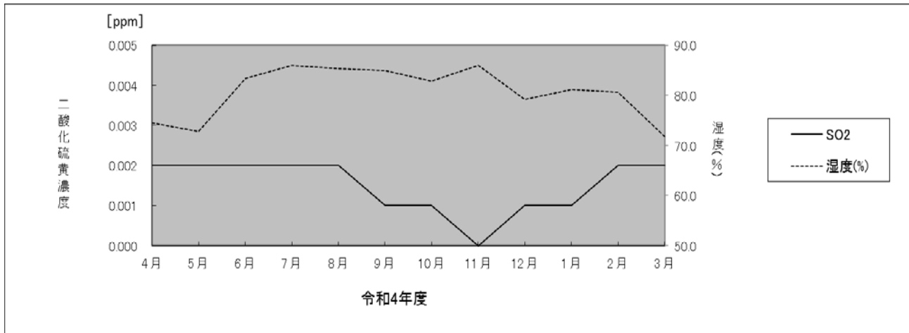
図3-1 二酸化硫黄濃度の季節的変動（市役所）
