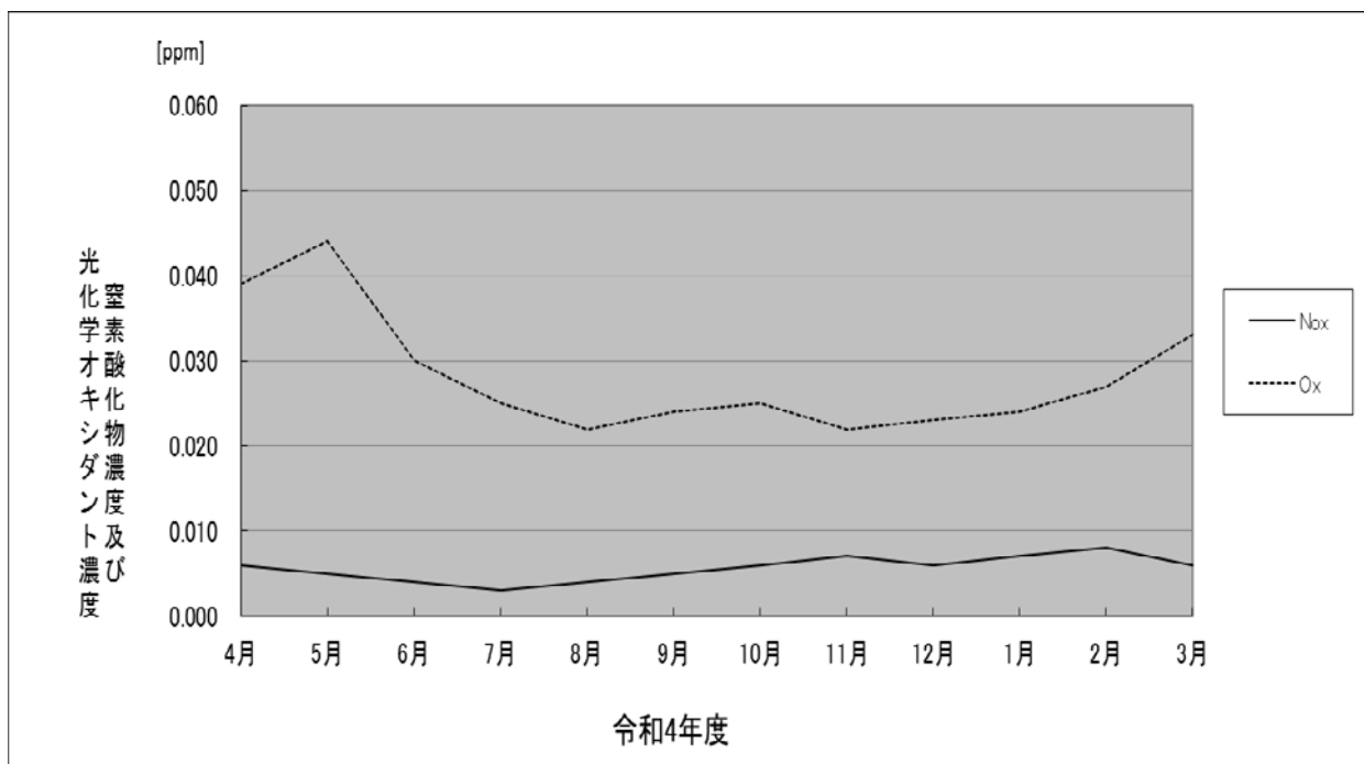
図3-7 窒素酸化物及び光化学オキシダント濃度の季節的変動
