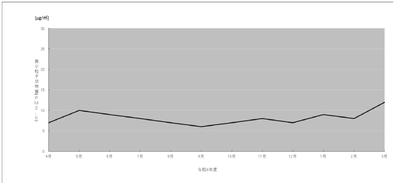
図3-8 微小粒子状物質(PM2.5)濃度の季節的変動
