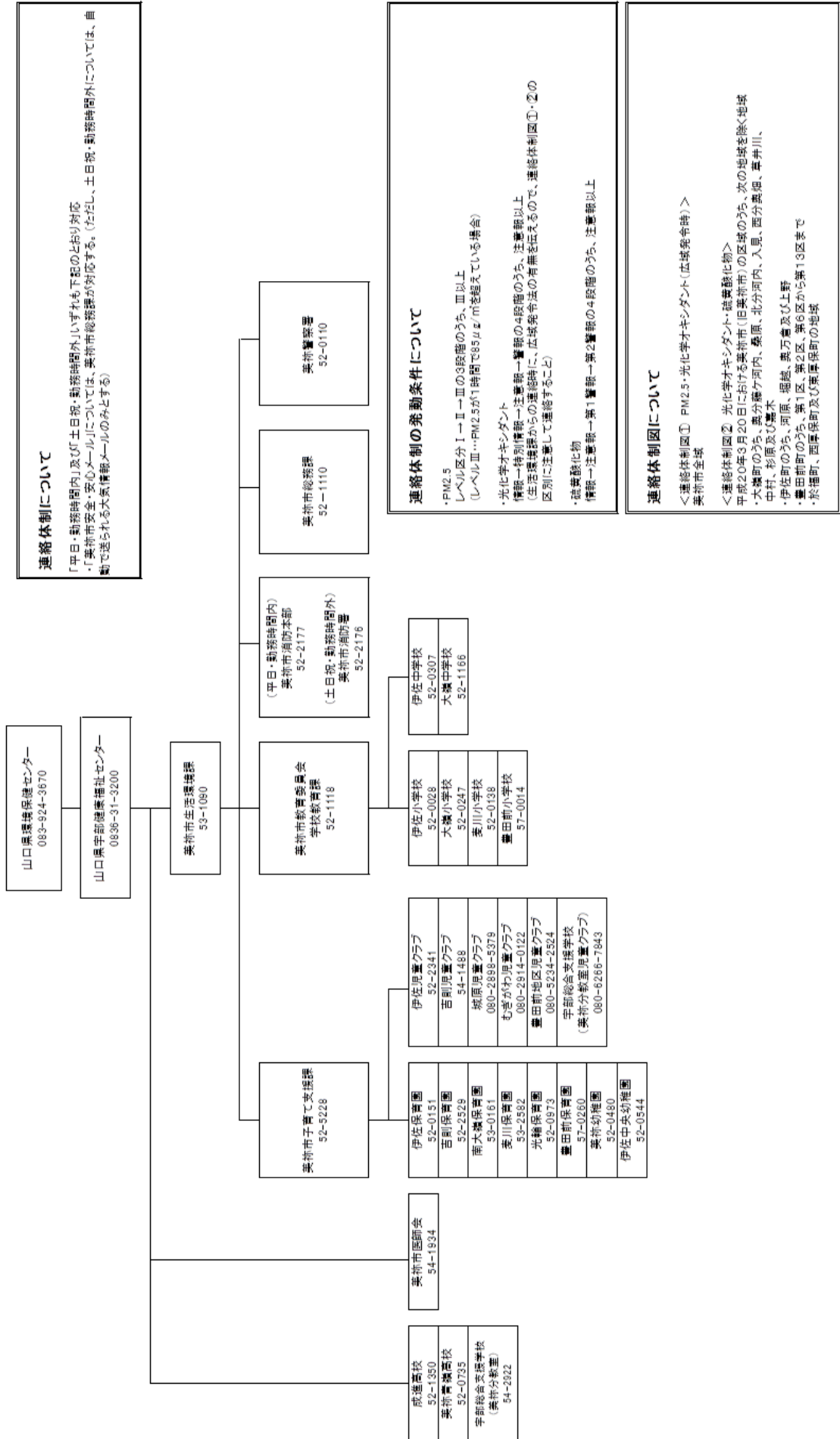
別図2 大気汚染連絡体制図 ※光化学オキシダント・硫黄酸化物 美林地域の一部地域限定
