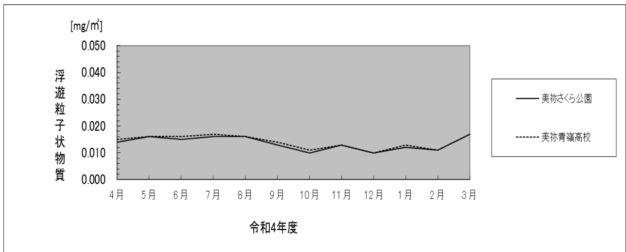
図3-2 浮遊粒子状物質濃度の季節的変動
