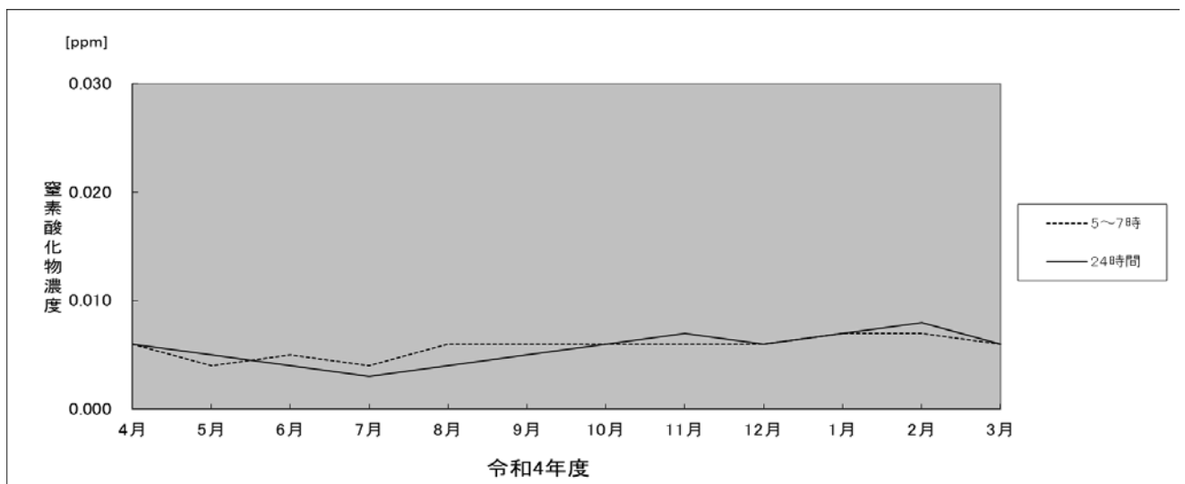
図 3-5 窒素酸化物濃度の季節的変動(24時間平均値と朝(5時~7時)の平均値との比較)
