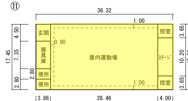
屋内運動場平面図
