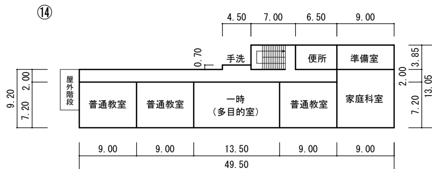
2階平面図
