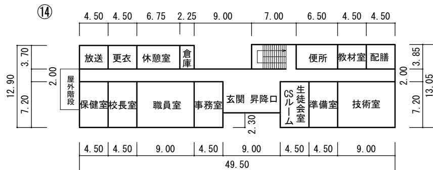
1階平面図
