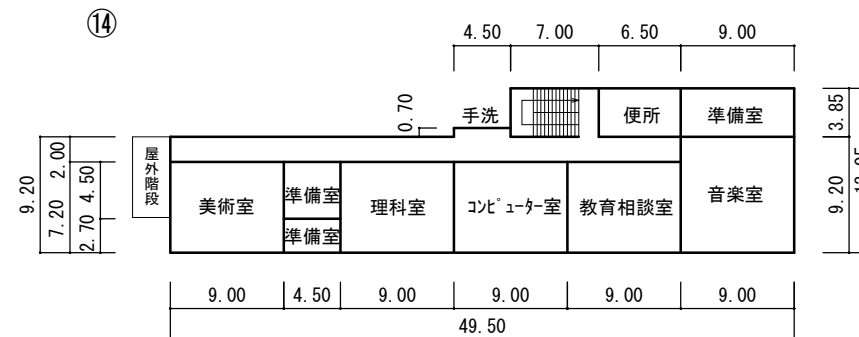
3階平面図
