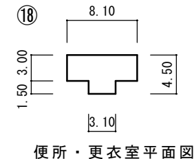
便所・更衣室平面図
