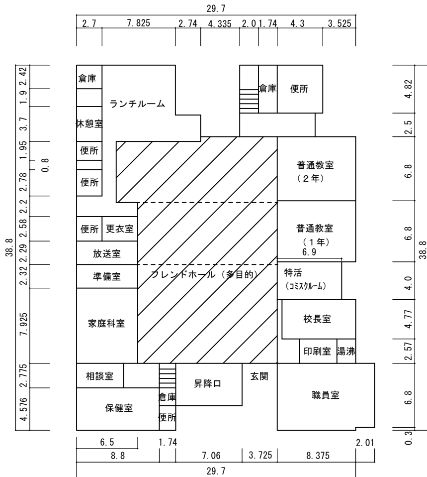
⑬教室棟 1 F
